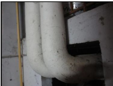
Photo N° 414 ECH-N°2 CALORIFUGEAGE --LOCAL CHAUFFERIE Conduits de fluide Laine minérale + enveloppe plâtrée
