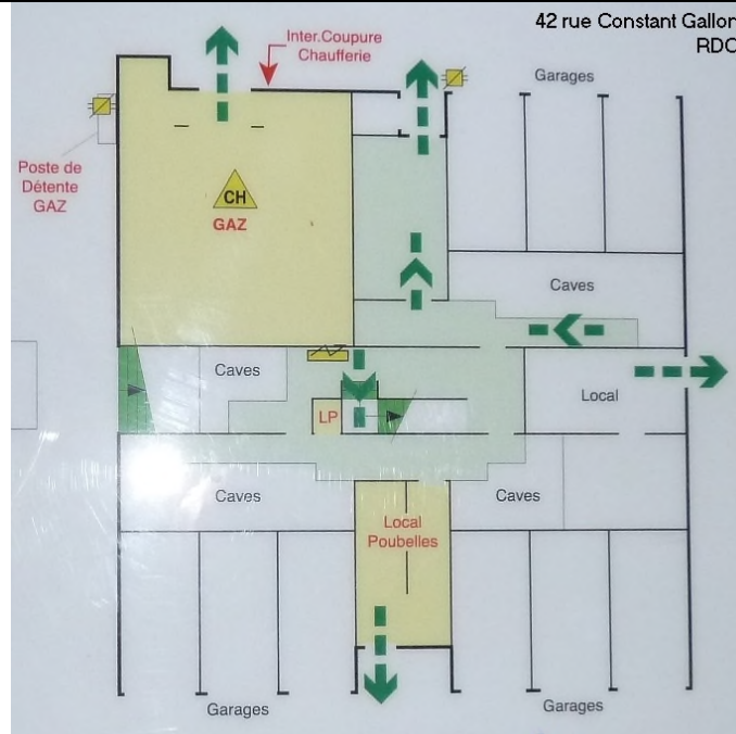
Planche (croquis) de repérage technique effectué par le cabinet : Cabinet Chambon-Levitan, auteur : LEVITAN Serge Dossier n° 13/IMO/0052/SLV du Adresse du bien : 42 rue Constant Gallon (Non communiqué) 77310 SAINT-FARGEAU-PONTHIERRY
