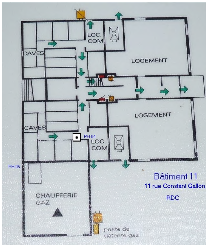
Planche (croquis) de repérage technique effectué par le cabinet : Cabinet Chambon-Levitan, auteur : LEVITAN Serge Dossier n° 13/IMO/0050/SLV du Adresse du bien : 11 rue Constant Gallon (Non communiqué) 77310 SAINT-FARGEAU-PONTHIERRY
