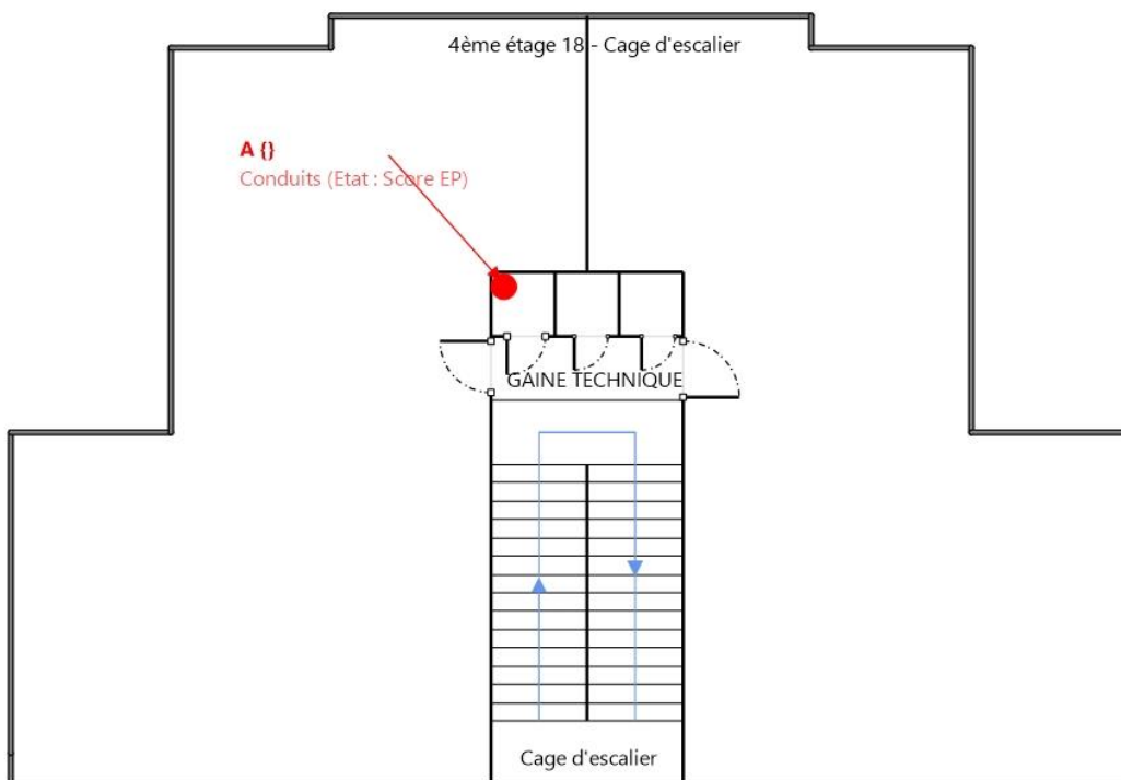
Planche (croquis) de repérage technique effectuée par le cabinet : ALLODIAGNOSTIC, auteur : Yann SYLVESTRE
