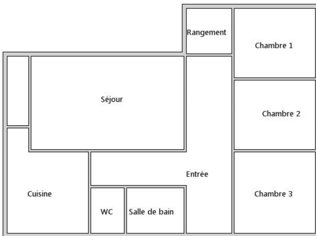
Planche (croquis) de repérage technique effectué par le cabinet : ALLODIAGNOSTIC, auteur : Jean-François RUBION Dossier n° 811405 du Adresse du bien : 23 RUE HENRI GUILLAUMET 478 47804B2347 77400 LAGNY SUR MARNE
