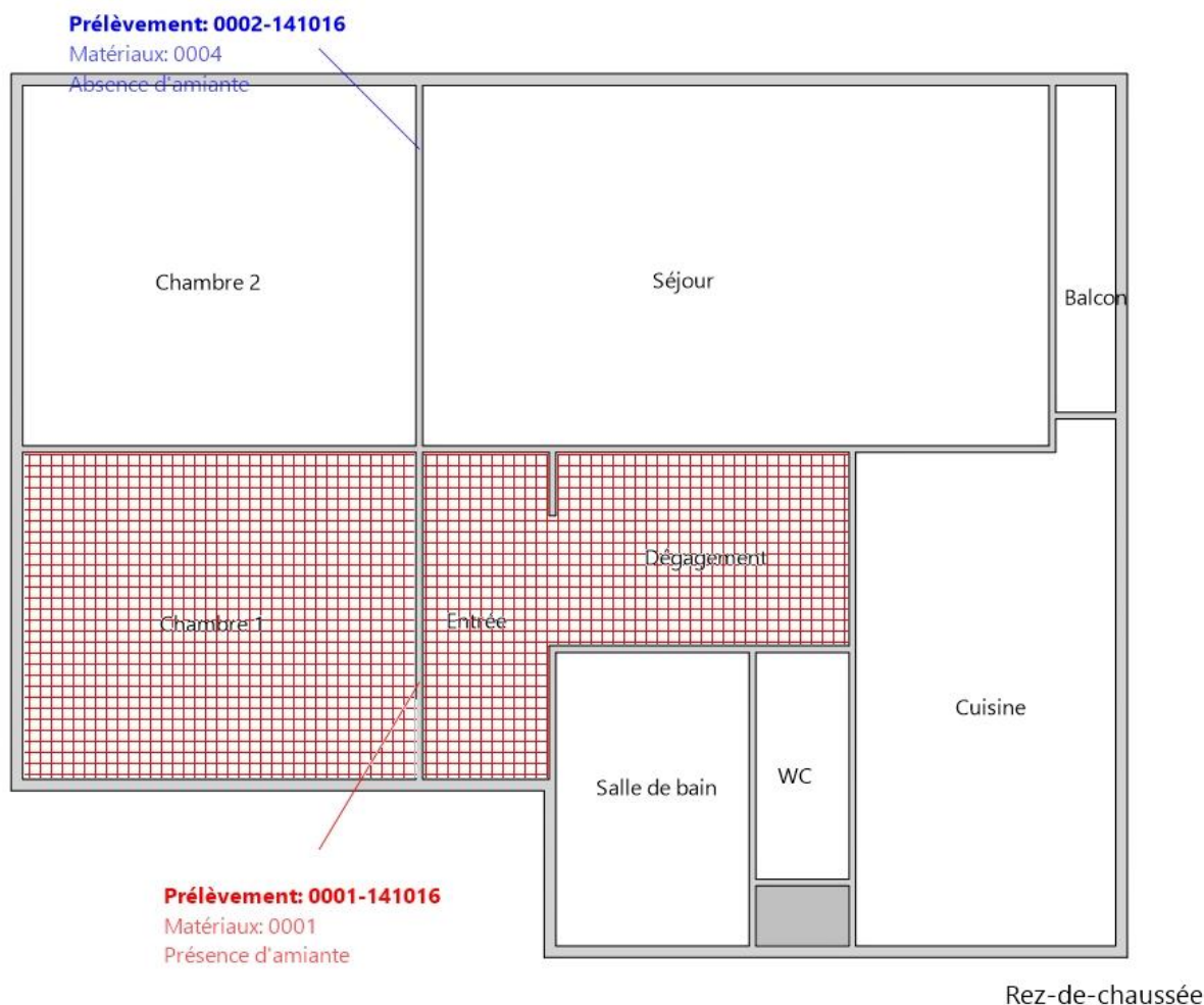
Planche (croquis) de repérage technique effectué par le cabinet : ALLODIAGNOSTIC, auteur : Boukhalafa SADALI Dossier n° 811671 du 14/10/2016 Adresse du bien : 18 ALLEE DES HETRES POURPRES 478 47805D0400 77400 LAGNY SUR MARNE
