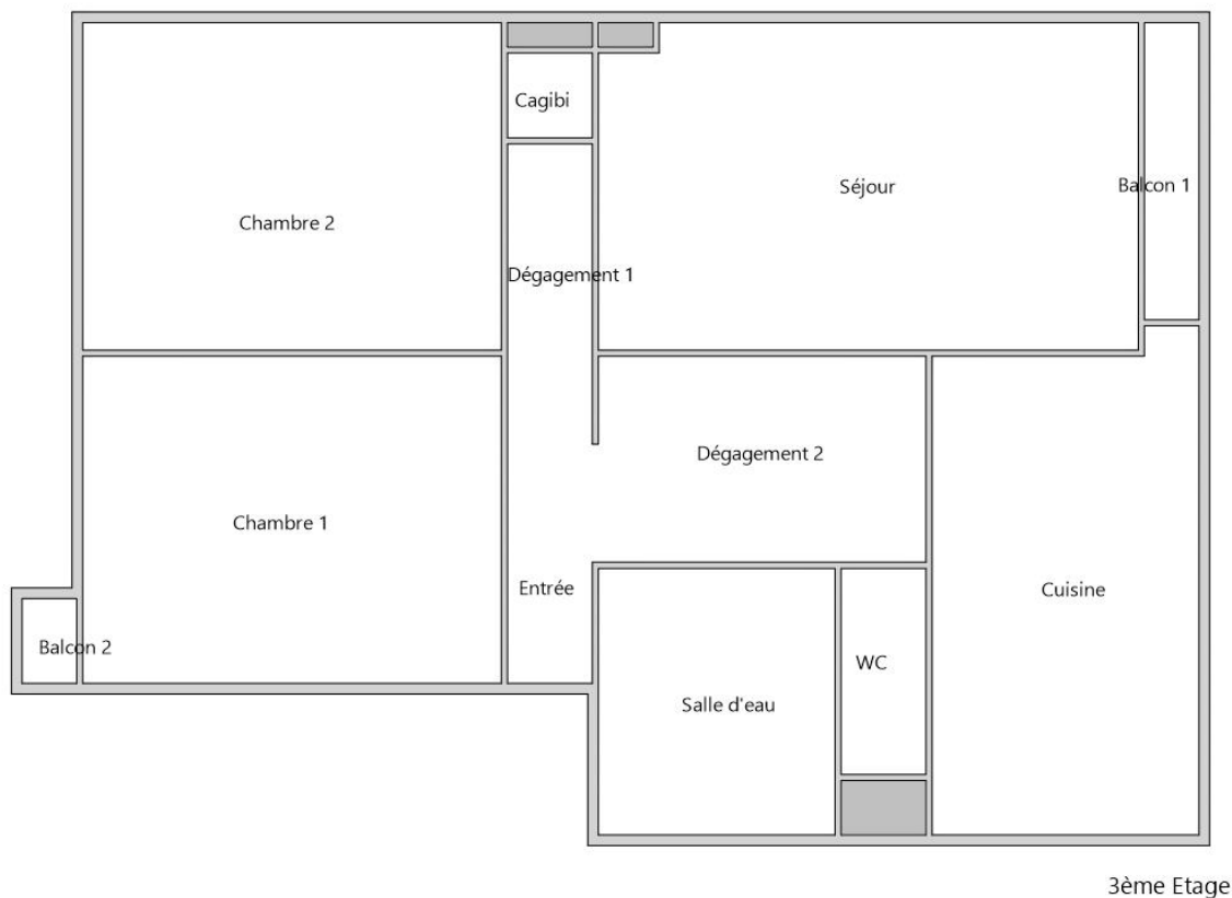
Planche (croquis) de repérage technique effectué par le cabinet : ALLODIAGNOSTIC, auteur : Boukhalfa SADALI Dossier n° 811953 du 21/10/2016 Adresse du bien : 18 RUE MARCEL RIVIERE 478 47807B3453 77400 LAGNY SUR MARNE
