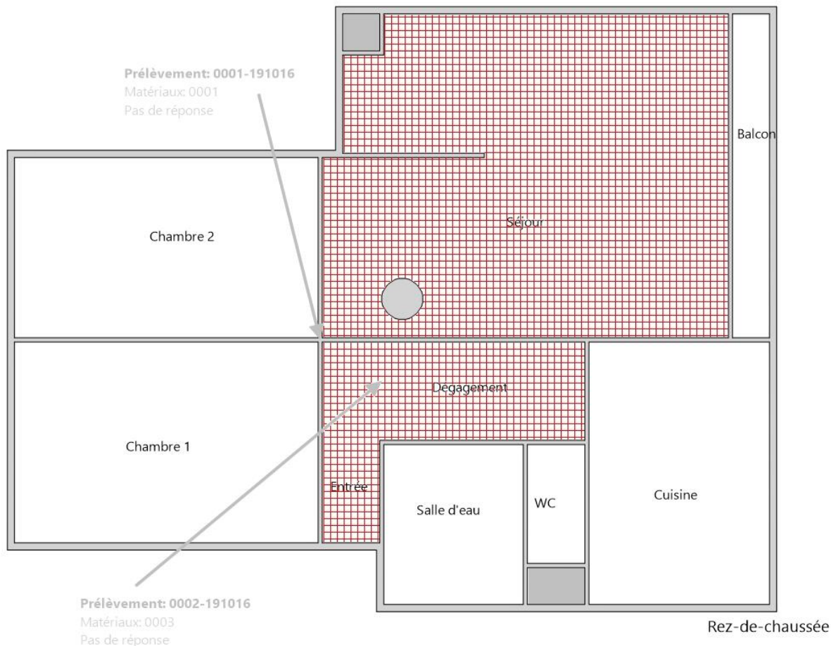
Planche (croquis) de repérage technique effectué par le cabinet : ALLODIAGNOSTIC, auteur : Boukhalafa SADALI Dossier n° 811947 du 19/10/2016 Adresse du bien : 8 ALLEE DES HETRES POURPRES 479 47907D0020 77400 LAGNY SUR MARNE
