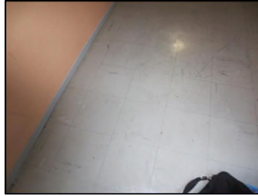
Photo N° 527 ECH-N°3 REVETEMENT DE SOL PALIER VOLEE ESCALIER 1 au12 Planchers Dalles de sol 30x30 avec colle noire
